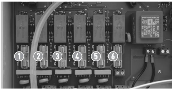
Abbildung 3: Feinsicherungen auf der Grundplatine
